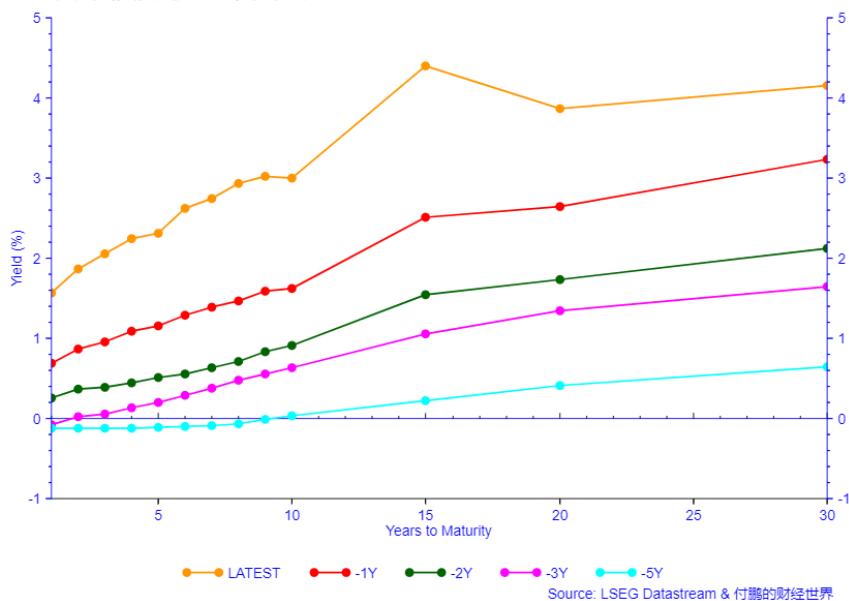
日本债券收益率曲线
